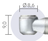
Cabeça: \varnothing 8,6 \text{ mm} Altura da Cabeça: 9,0 mm
